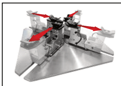
grande table de fixation pour une prise jusqu'à 24" de diamètre de jante
