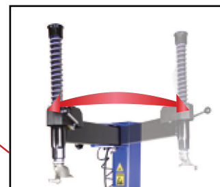
bras de montage à pivotement latéral
