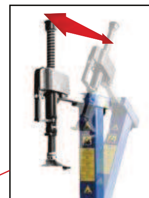
robuste colonne basculante pneumatique
